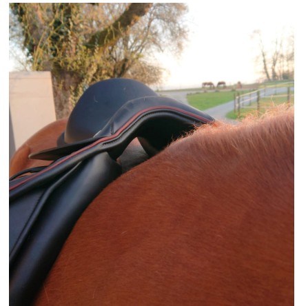
Foto von vorne seitlich in den Kissenkanal, Sattel ohne Unterlage, gegurtet
